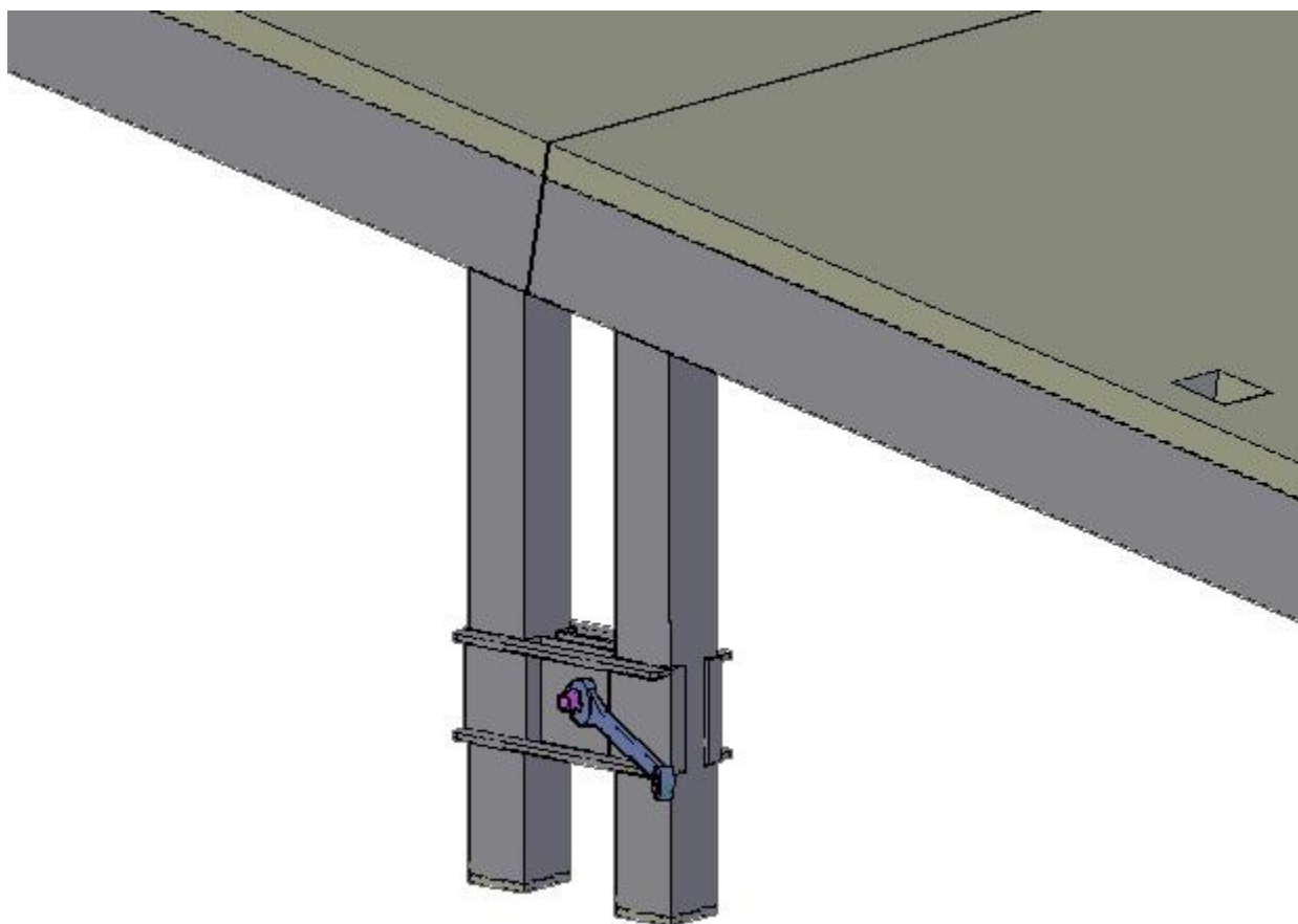
Detalle de unión entre patas de los módulos rampa
